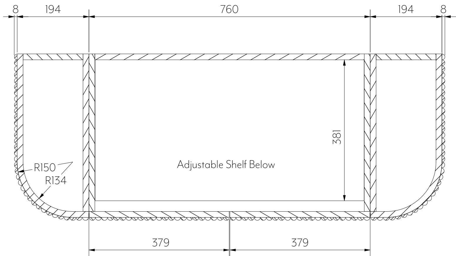
Section A-A
